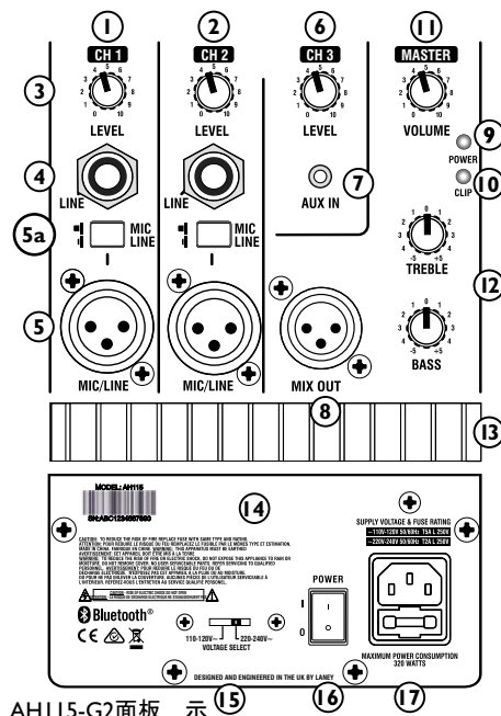
AH I15-G2面板 示
